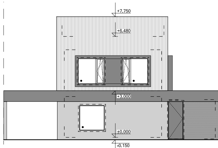
JIŽNÍ POHLED
