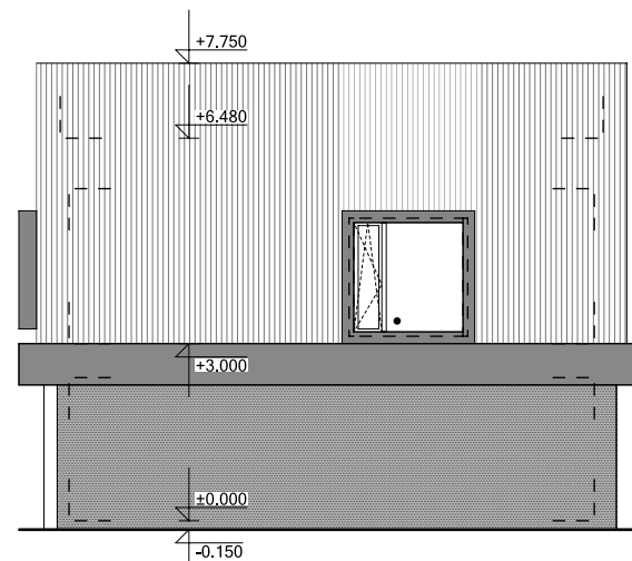
VÝCHODNÍ POHLED
