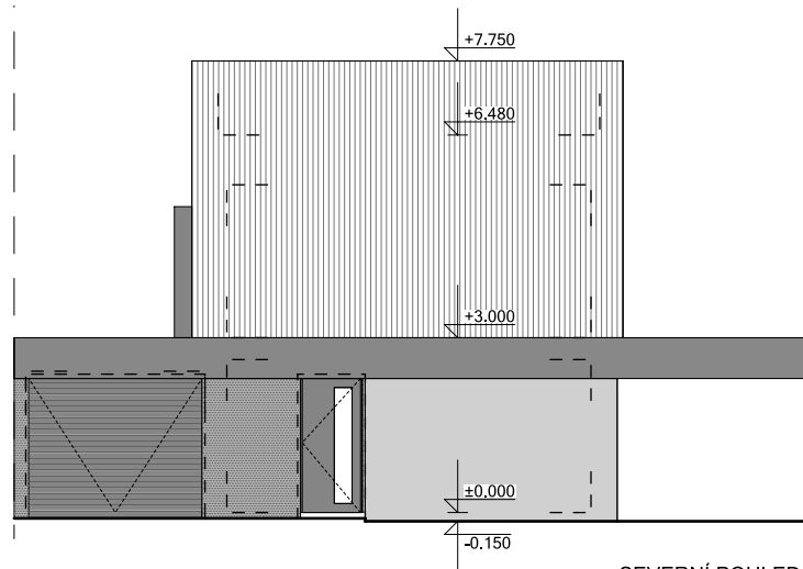
SEVERNÍ POHLED
